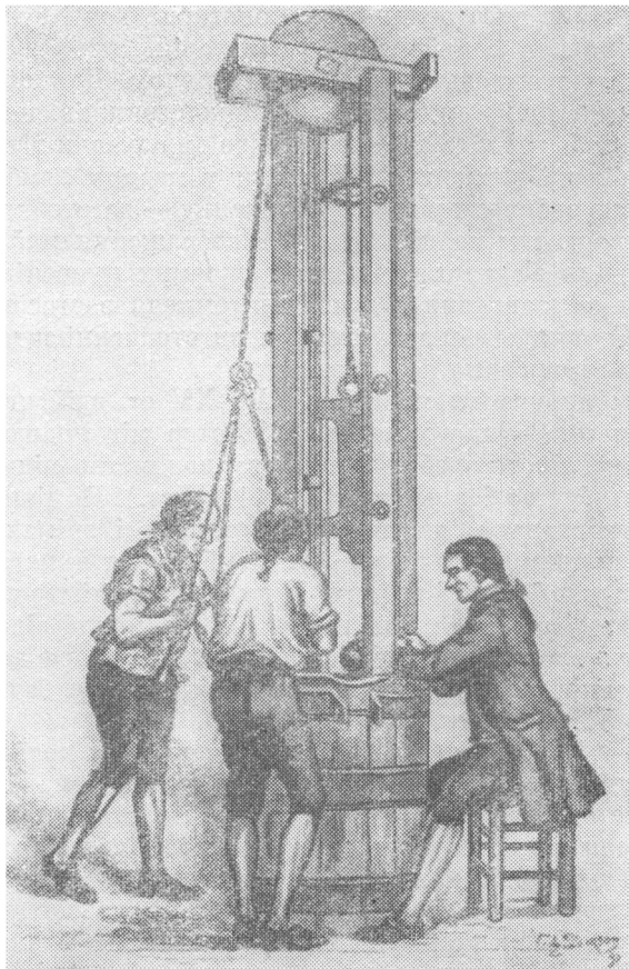
Механічний молот, що застосовувався на монетарнях XV—XVII ст.
